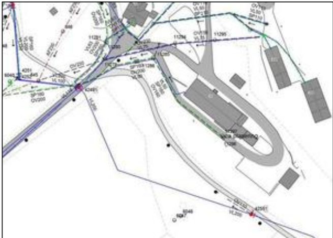
Figur 34: Ledningskart som viser eksisterende VA-infrastruktur.
